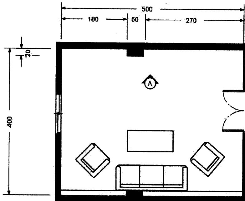
平面圖 單位：cm
